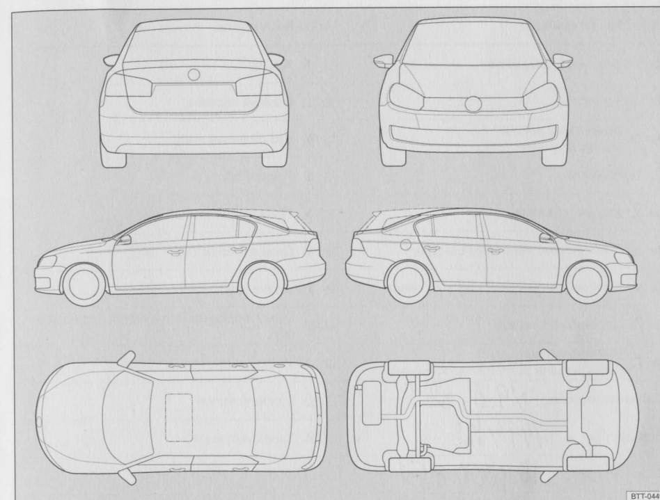
Obr. 7 Schematické zobrazení. Platí pro všechna vozidla a formy karoserie.
