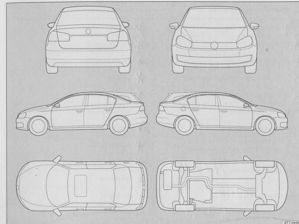
Abb. 10 Prinzipdarstellung. Gilt für alle Fahrzeuge und Karosserieformen.
